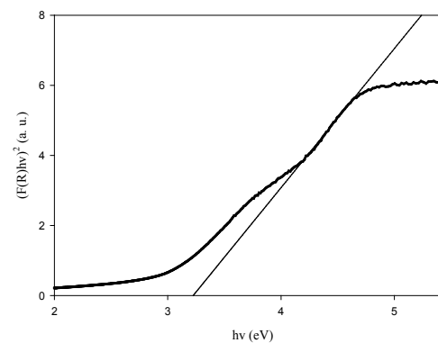
(d) E'_{opt} = 3.23 \text{ eV}
